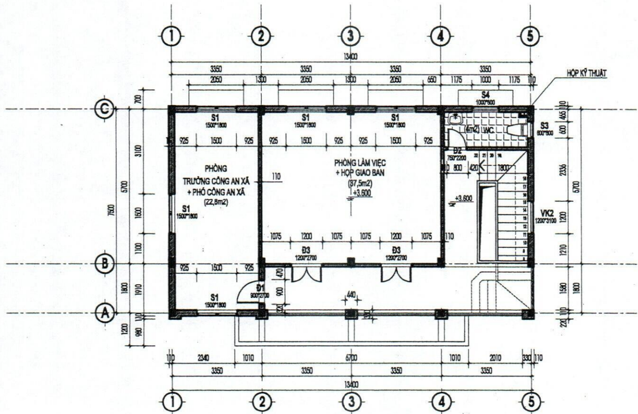
MẶT BẰNG TẦNG 2
